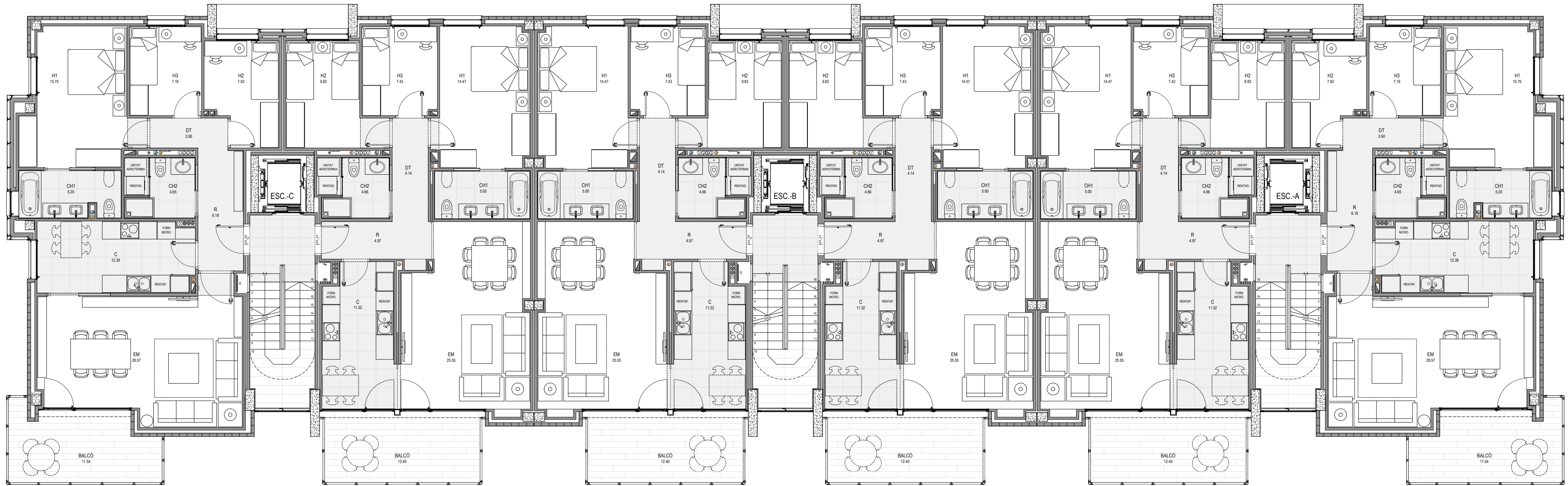
PLANTA TIPUS
